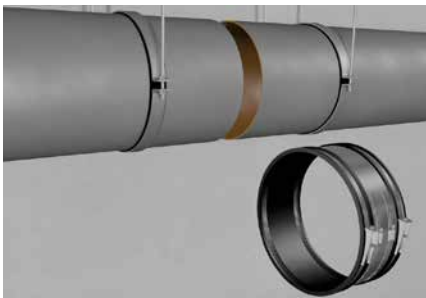
Rohrspitzenden ausrichten.
